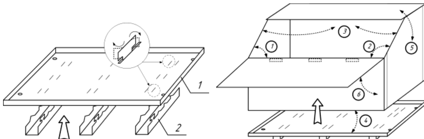
Рис. 2 Рекомендуемый порядок сборки ящика для песка
